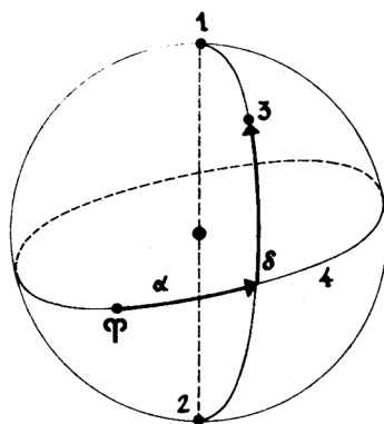
Рис. 4.1. Экваториальная система координат: 1,2 — соответственно северный и южный полюсы мира; 3 — светило; 4 — экватор
