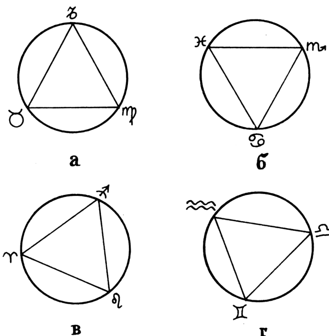
Рис. 5.2. Тригоны: а — Земли; б — Воды; в — Огня; г — Воздуха
