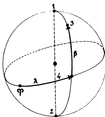
Рис. 4.2. Эклиптическая система координат: 1, 2 — соответственно северный и южный полюсы эклиптики; 3 — светило; 4 — эклиптика
