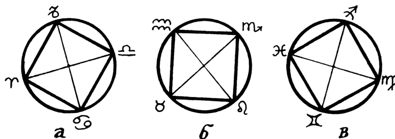
Рис. 5.4. Кресты: а — кардинальный; б — фиксированный; в — мутабельный
