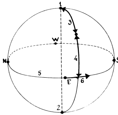
Рис. 4.3. Горизонтальная система координат: 1 — зенит; 2 — надир; 3 — зенитное расстояние; 4 — высота; 5 — линия горизонта; 6 — азимут
