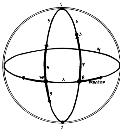
Рис. 5.1. Географическая система координат: 1,2 — северный и южный полюсы; 3 — Москва; 5 — экватор; 5 — Гринвичский меридиан; 6 — меридиан
