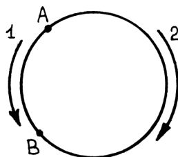
Рис. 6.5. Расстояния на окружности: 1, 2 — малая и большая дуги
