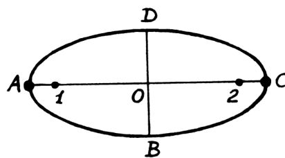
Рис. 4.4. Эллипс: 1,2 — фокусы эллипса (если Солнце в фокусе 1, то точка A — перигелий, точка C — афелий); AO — большая полуось; BO — малая полуось
