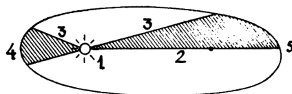
Рис. 3.2. Иллюстрация второго закона Кеплера (заштрихованные площади равны): 1,2 — первый и второй фокусы; 3 — радиус-вектор; 4 — перигелий; 5 — афелий
