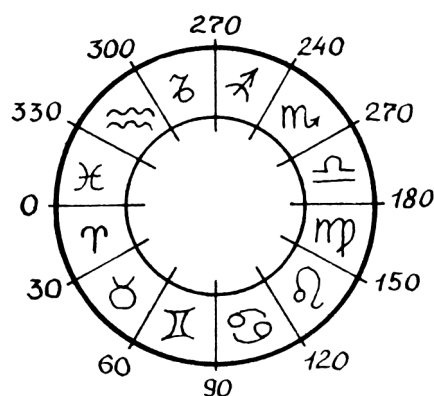
Рис. 4.6. Градуальный круг Зодиака
