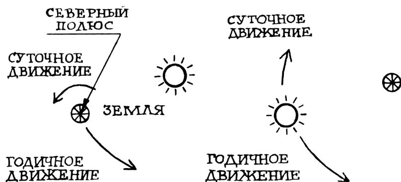
Рис. 4.7. Годичное и суточное движение Солнца относительно Земли
