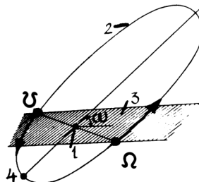
Рис. 4.5. Узлы орбиты планет: 1 — Солнце; \omega — угол наклона плоскости орбиты планеты 2 к плоскости эклиптики 3; 4 — перигелий
